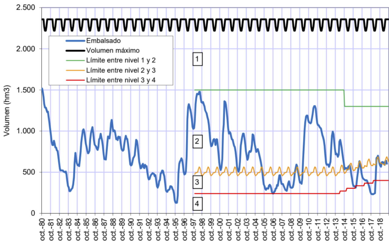
Figura 1 "Niveles característicos y volúmenes reales embalsados a primeros de mes en el sistema Entrepeñas-Buendía desde el comienzo de la operación del ATS" del Informe de situación de la Comisión Central de explotación del ATS de julio de 2019
