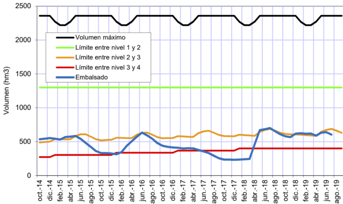
Figura 3 "Niveles característicos y volúmenes embalsados a primeros de mes en el sistema Entrepeñas-Buendía desde octubre de 2014" del Informe de situación de la Comisión Central de explotación del ATS de julio de 2019
