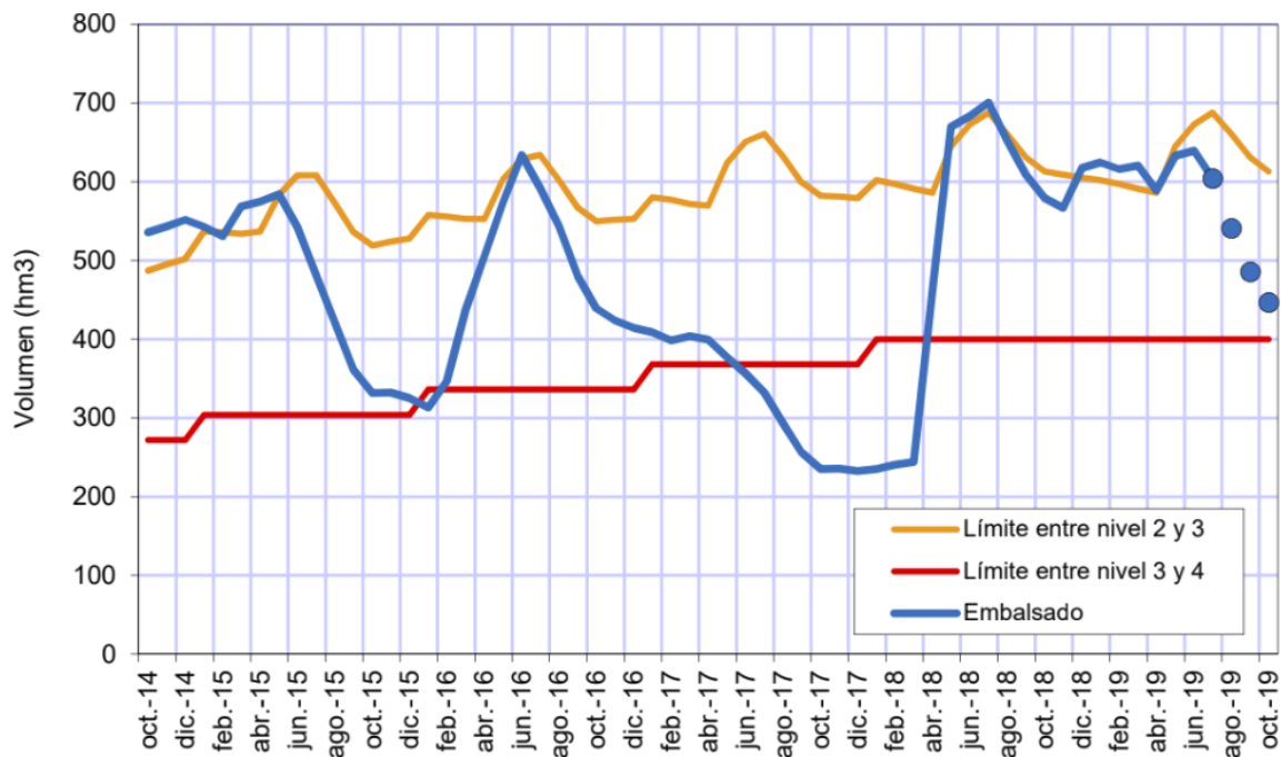
Figura 7 "Evolución de las reservas en Entrepeñas-Buendía y previsión para los próximos tres meses" del Informe de situación de la Comisión Central de explotación del ATS de julio de 2019
